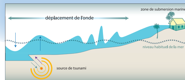
Formation d'un tsunami modifié d'après M. Péroche, DEAL 2016
