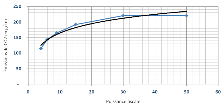
Figure 15 - Courbe de tendance des émissions de CO 2 en fonction de la puissance fiscale des voitures diesel en vente en 2010
