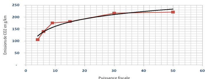
Figure 15 - Courbe de tendance des émissions de CO 2 en fonction de la puissance fiscale des voitures diesel en vente en 2010
