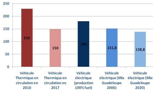
Figure 20 -Emission de CO 2 des véhicules électriques en fonction de la source d'énergie
