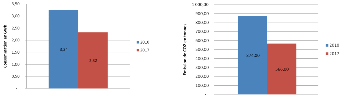
Figure 19 - Comparaison entre les consommations énergétiques et les émissions de CO 2 du parc de véhicules particuliers entre 2010 et 2017
