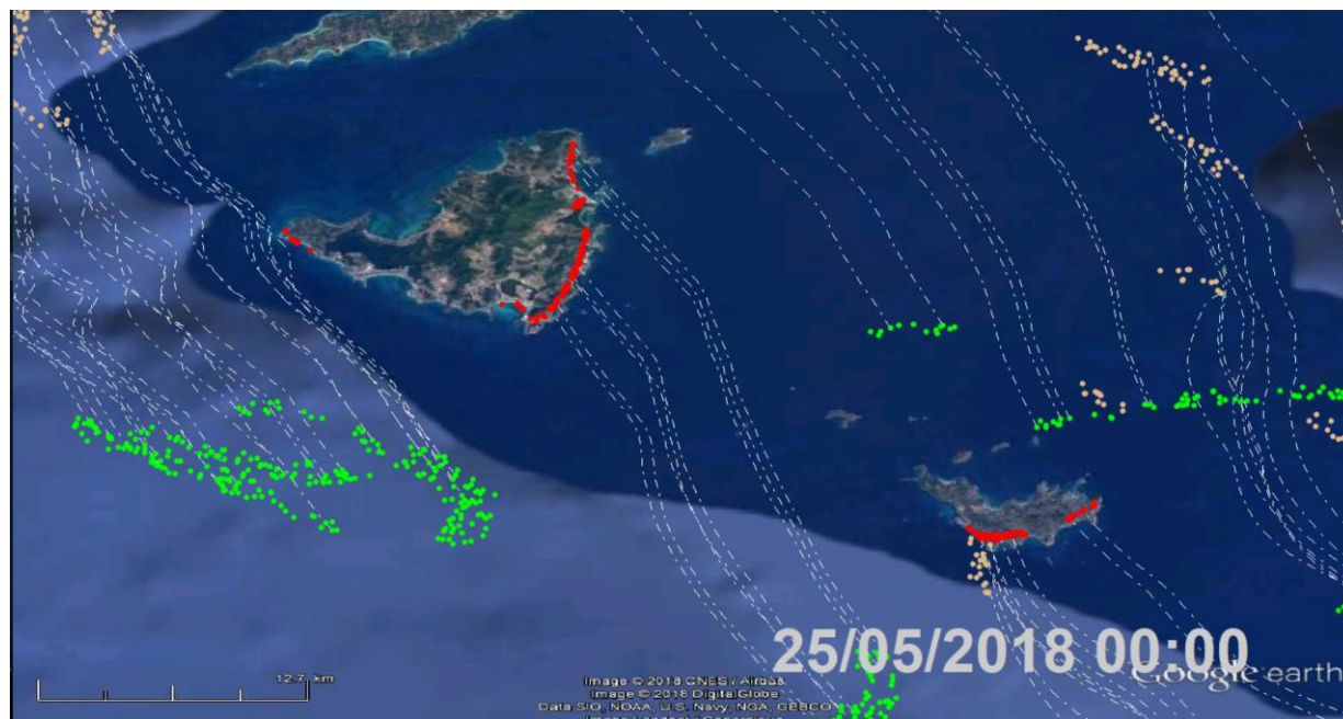
Figure 8 Radeaux de sargasses, positions de détection (points verts), trajectoires (pointillés blancs), positions le 25/05/2018 à 00:00 (heure locale) et positions d'échouages prévues (points rouges) sur Saint-Martin et Saint-Barthélemy.
