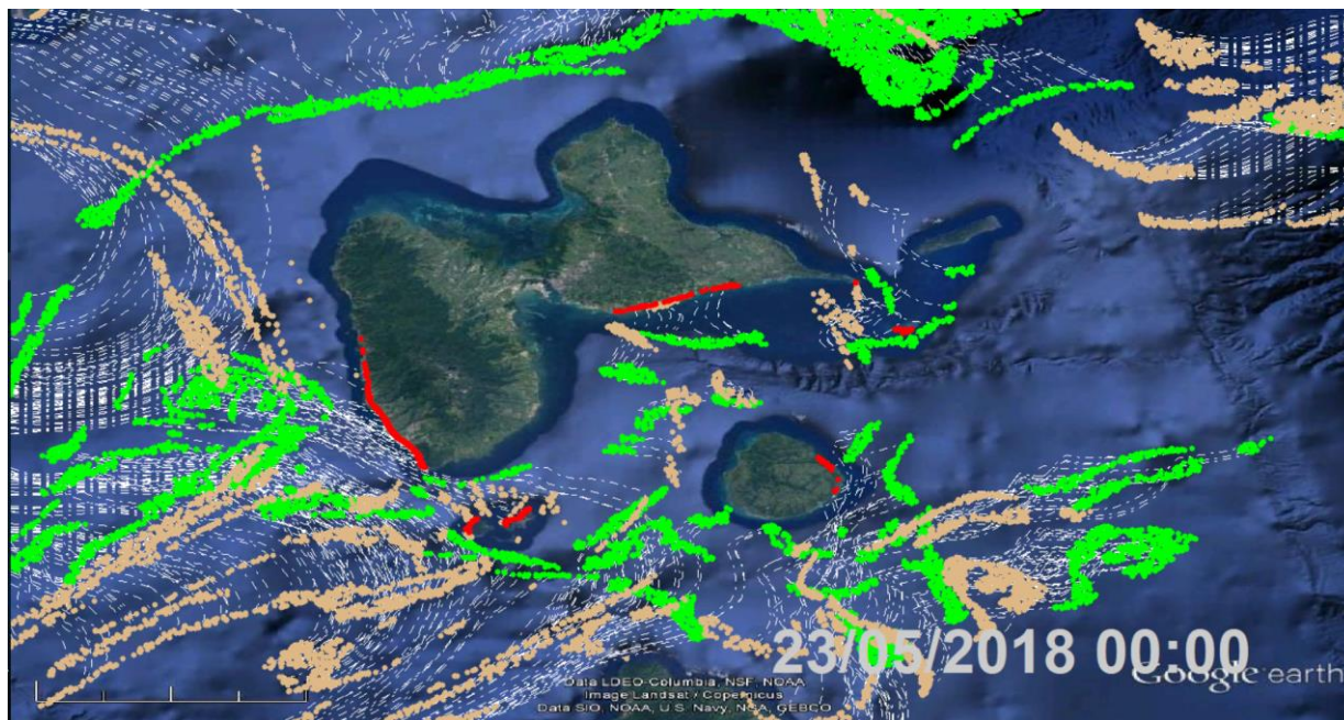
Figure 2 Radeaux de sargasses, positions de détection (points verts), trajectoires (pointillés blancs), positions le 23/05/2018 à 00:00 (heure locale) et positions d'échouages prévues (points rouges) sur la Guadeloupe.
