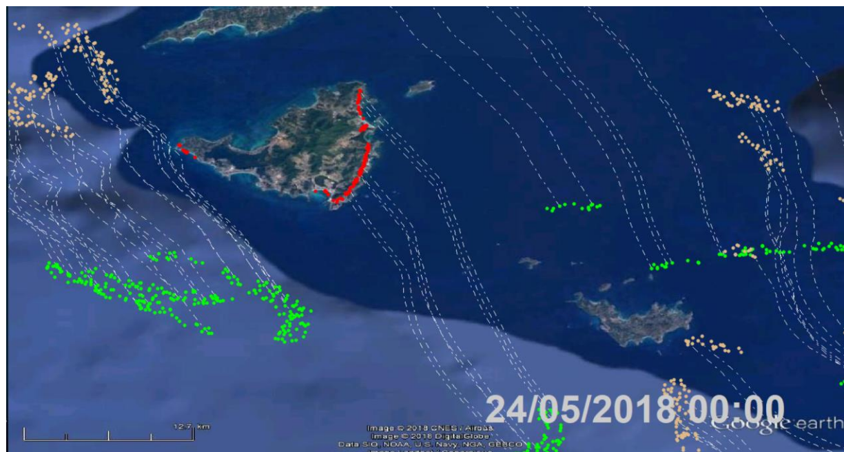
Figure 7 Radeaux de sargasses, positions de détection (points verts), trajectoires (pointillés blancs), positions le 24/05/2018 à 00:00 (heure locale) et positions d'échouages prévues (points rouges) sur Saint-Martin et Saint-Barthélemy.
