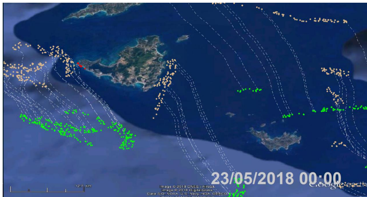
Figure 6 Radeaux de sargasses, positions de détection (points verts), trajectoires (pointillés blancs), positions le 23/05/2018 à 00:00 (heure locale) et positions d'échouages prévues (points rouges) sur Saint-Martin et Saint-Barthélemy.
