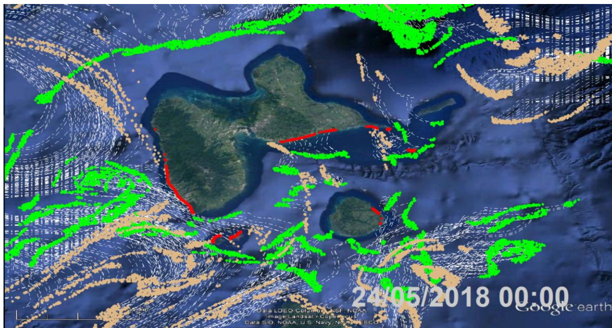
Figure 3 Radeaux de sargasses, positions de détection (points verts), trajectoires (pointillés blancs), positions le 24/05/2018 à 00:00 (heure locale) et positions d'échouages prévues (points rouges) sur la Guadeloupe.
