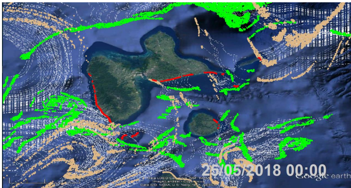
Figure 4 Radeaux de sargasses, positions de détection (points verts), trajectoires (pointillés blancs), positions le 25/05/2018 à 00:00 (heure locale) et positions d'échouages prévues (points rouges) sur la Guadeloupe.
