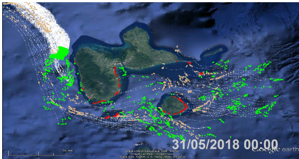
Figure 3 Radeaux de sargasses, positions de détection (points verts), trajectoires (pointillés blancs), positions le 31/05/2018 à 00:00 (heure locale) et positions d'échouages prévues (points rouges) sur la Guadeloupe.
