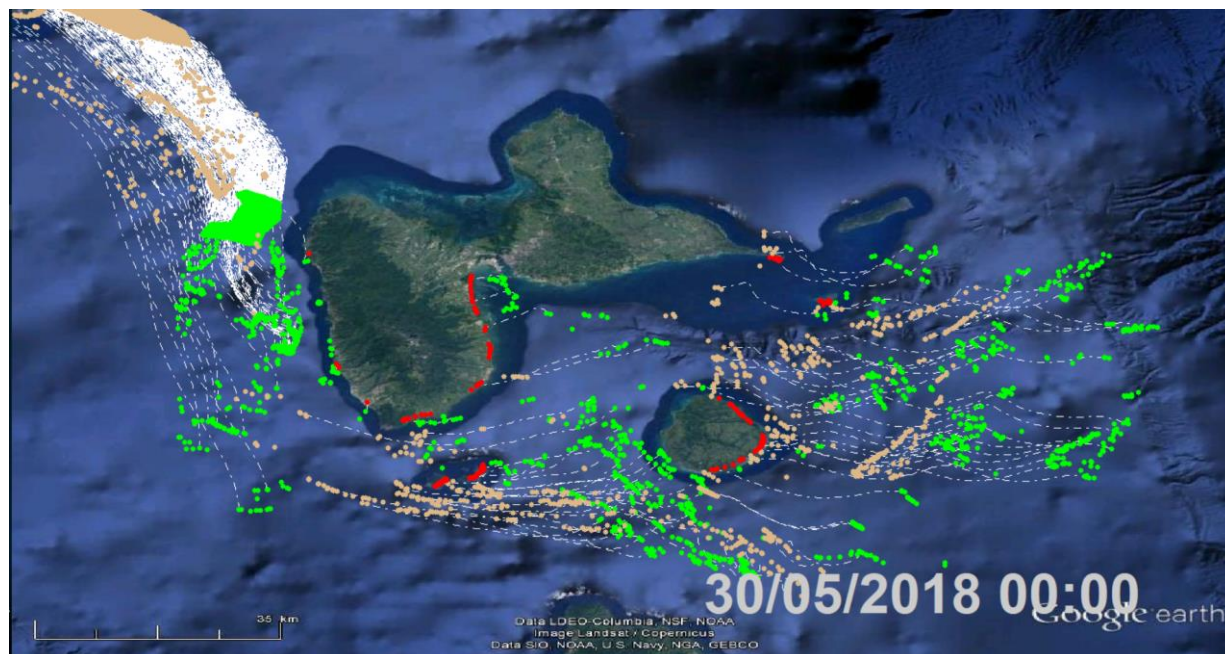
Figure 2 Radeaux de sargasses, positions de détection (points verts), trajectoires (pointillés blancs), positions le 30/05/2018 à 00:00 (heure locale) et positions d'échouages prévues (points rouges) sur la Guadeloupe.
