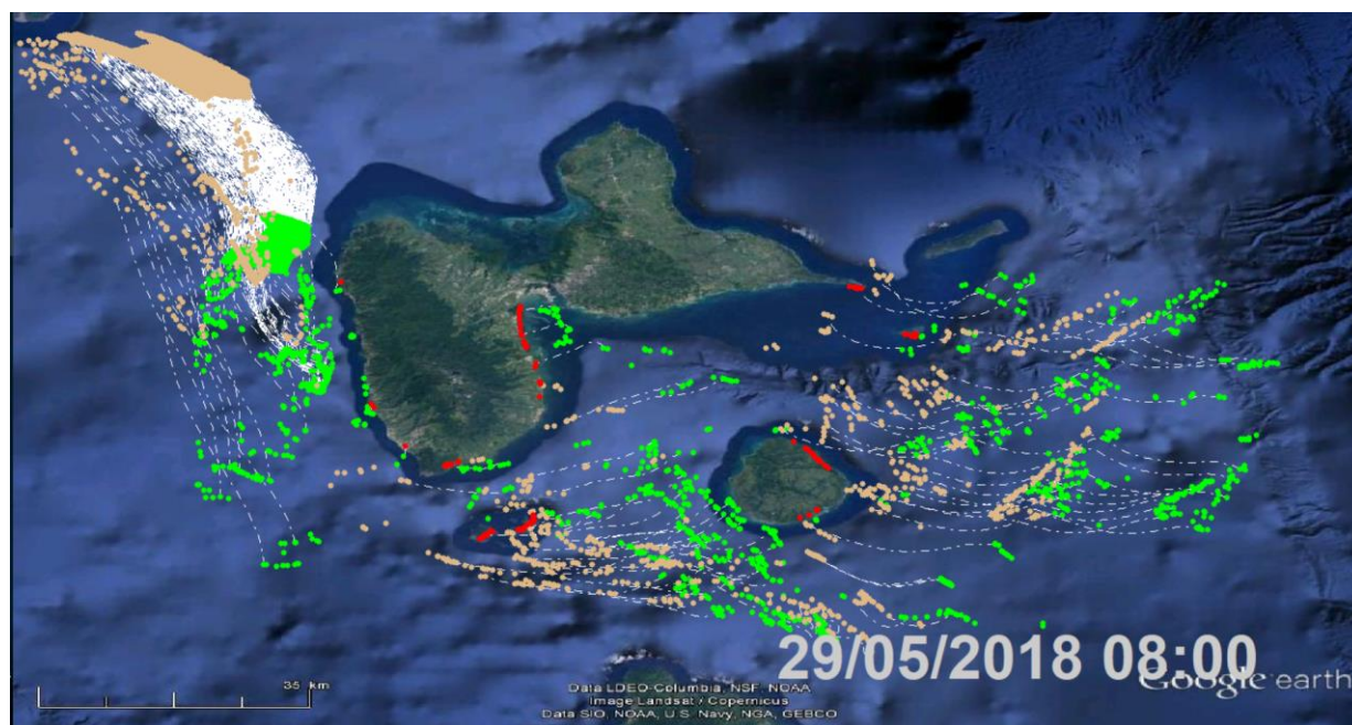
Figure 1 Radeaux de sargasses, positions de détection (points verts), trajectoires (pointillés blancs), positions le 29/05/2018 à 08:00 (heure locale) et positions d'échouages prévues (points rouges) sur la Guadeloupe.
