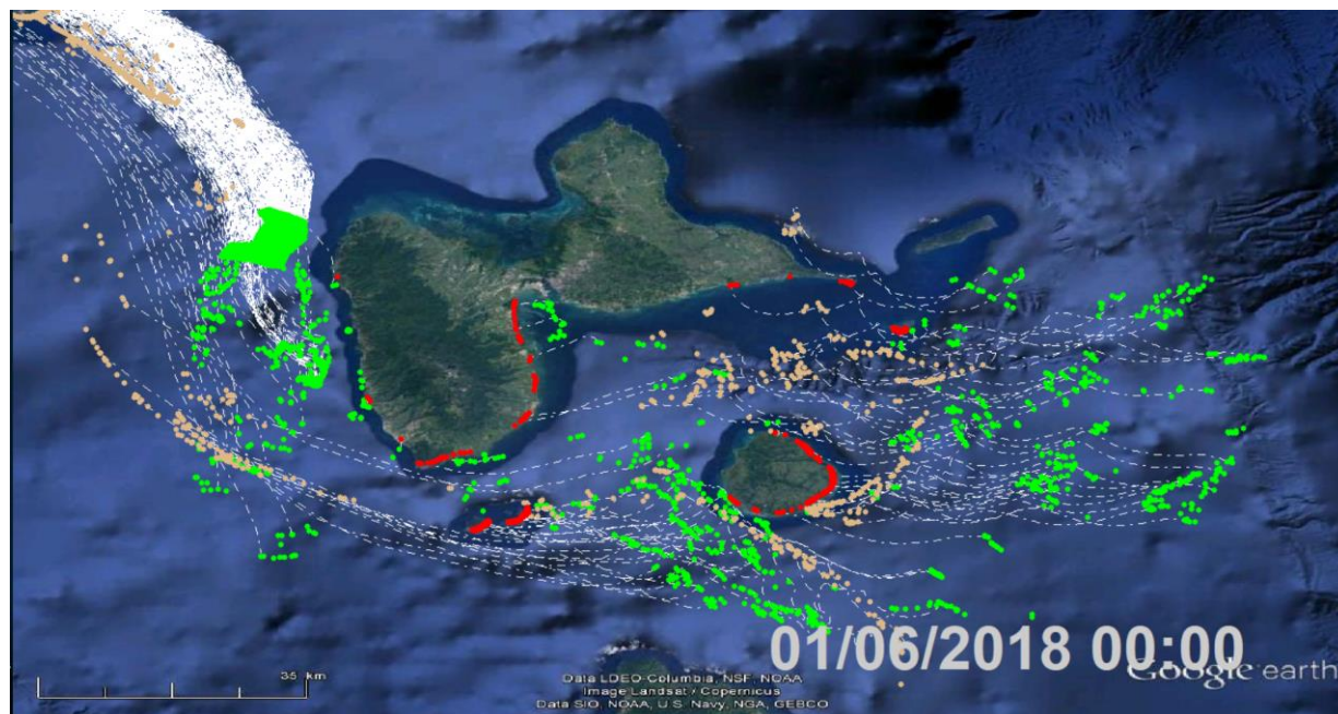
Figure 4 Radeaux de sargasses, positions de détection (points verts), trajectoires (pointillés blancs), positions le 01/06/2018 à 00:00 (heure locale) et positions d'échouages prévues (points rouges) sur la Guadeloupe.
