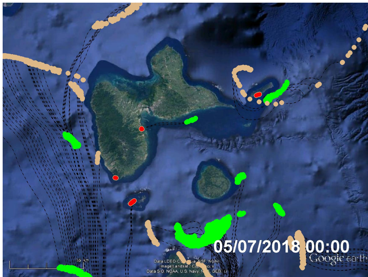
Figure 3 Radeaux de sargasses, positions de détection (points verts), trajectoires (pointillés blancs), positions le 05/07/2018 à 00:00 (heure locale) et positions d'échouages prévues (points rouges) sur la Guadeloupe.
