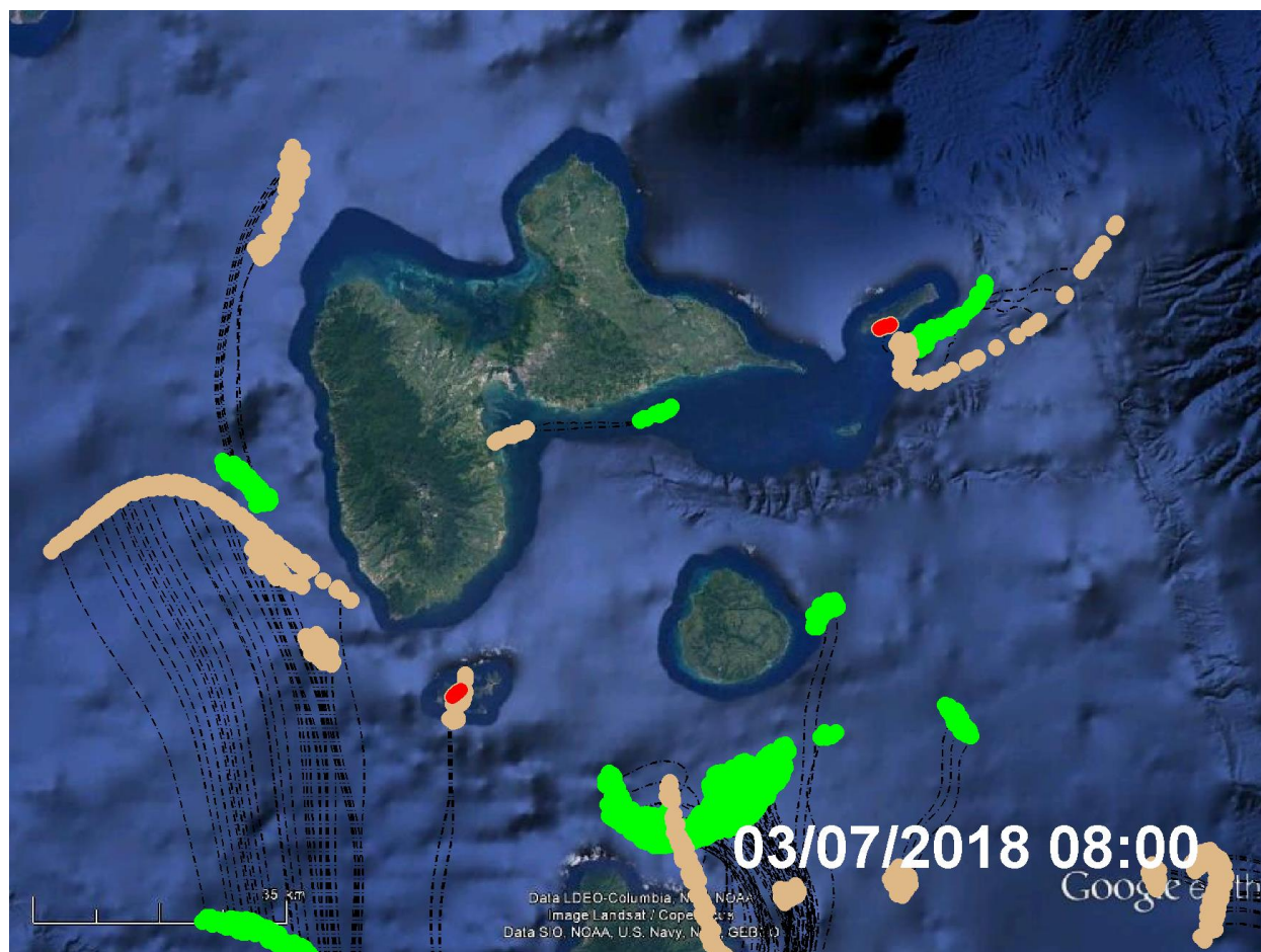
Figure 1 Radeaux de sargasses, positions de détection (points verts), trajectoires (pointillés blancs), positions le 03/07/2018 à 08:00 (heure locale) et positions d'échouages prévues (points rouges) sur la Guadeloupe.
