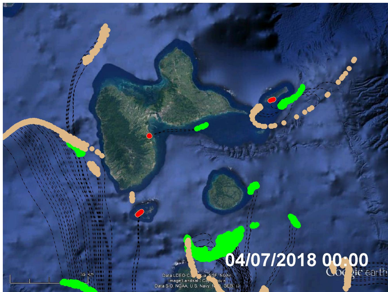
Figure 2 Radeaux de sargasses, positions de détection (points verts), trajectoires (pointillés blancs), positions le 04/07/2018 à 00:00 (heure locale) et positions d'échouages prévues (points rouges) sur la Guadeloupe.
