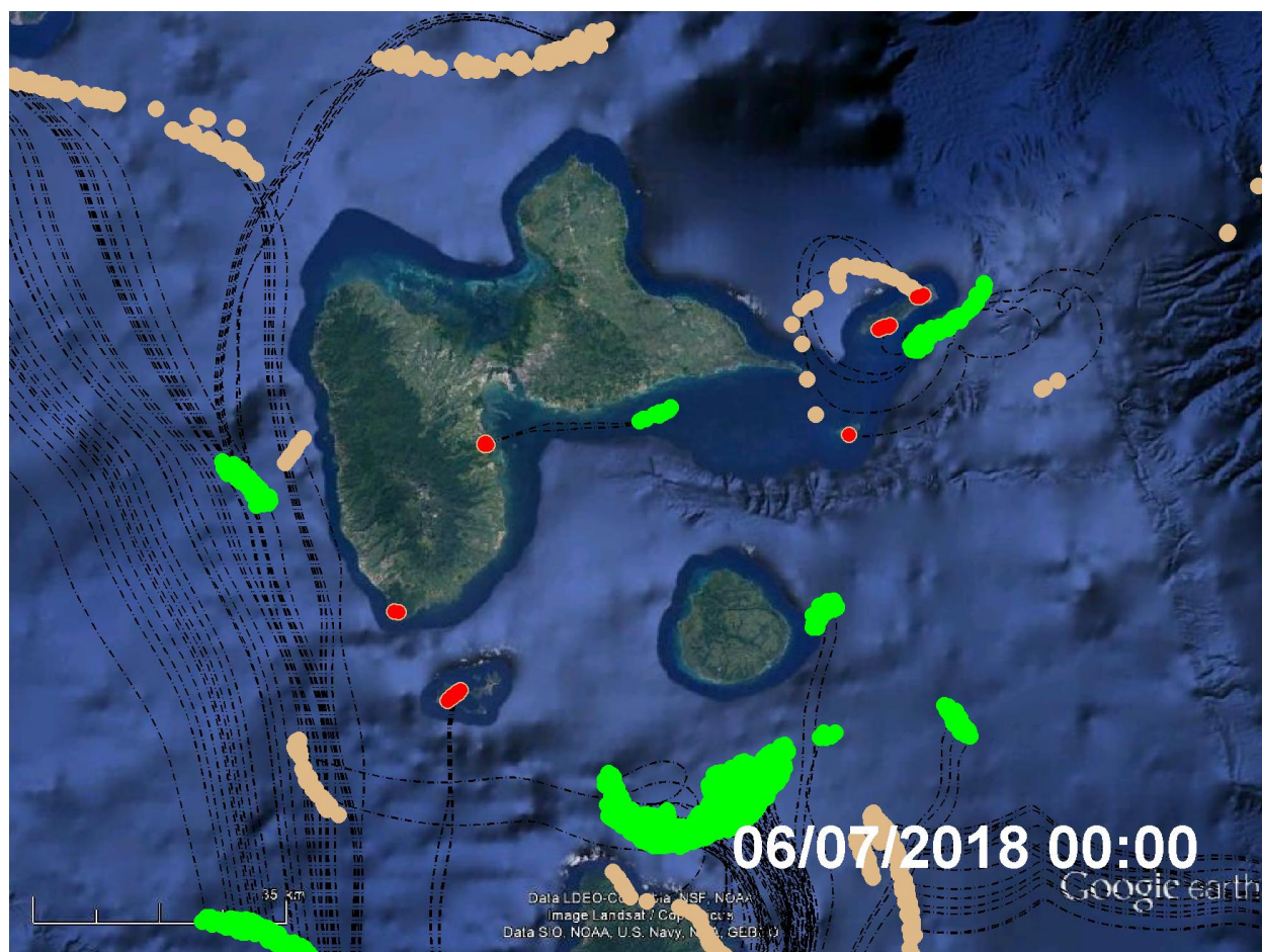
Figure 4 Radeaux de sargasses, positions de détection (points verts), trajectoires (pointillés blancs), positions le 06/07/2018 à 00:00 (heure locale) et positions d'échouages prévues (points rouges) sur la Guadeloupe.
