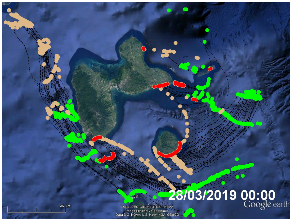
Figure 3 Radeaux de sargasses, positions de détection (points verts), trajectoires (pointillés blancs), positions le 28/03/2019 à 00:00 (heure locale) et positions d'échouages prévues (points rouges) sur la Guadeloupe.
