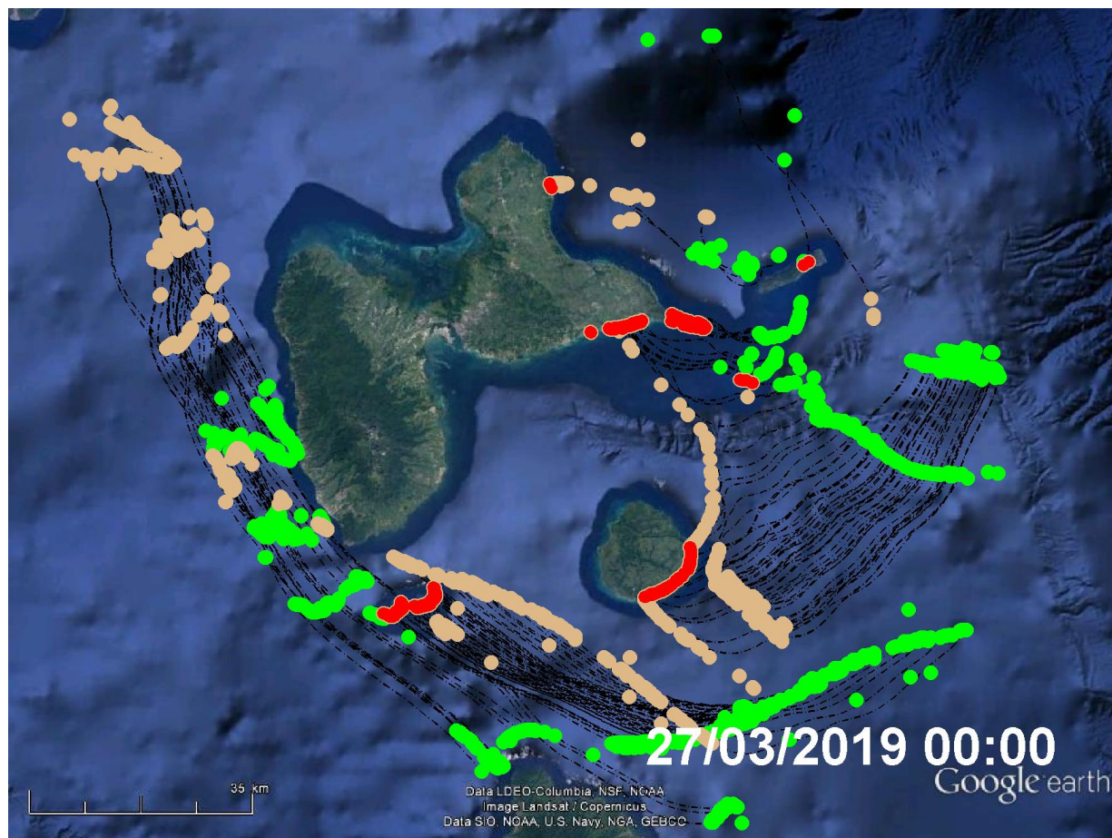
Figure 2 Radeaux de sargasses, positions de détection (points verts), trajectoires (pointillés blancs), positions le 27/03/2019 à 00:00 (heure locale) et positions d'échouages prévues (points rouges sur la Guadeloupe).
