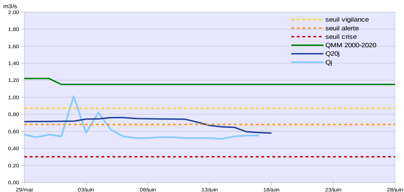
Courbe 3 : Variation du débit moyen sur 20 jours en 2024 sur la Rivière Moustique à Petit-Bourg
