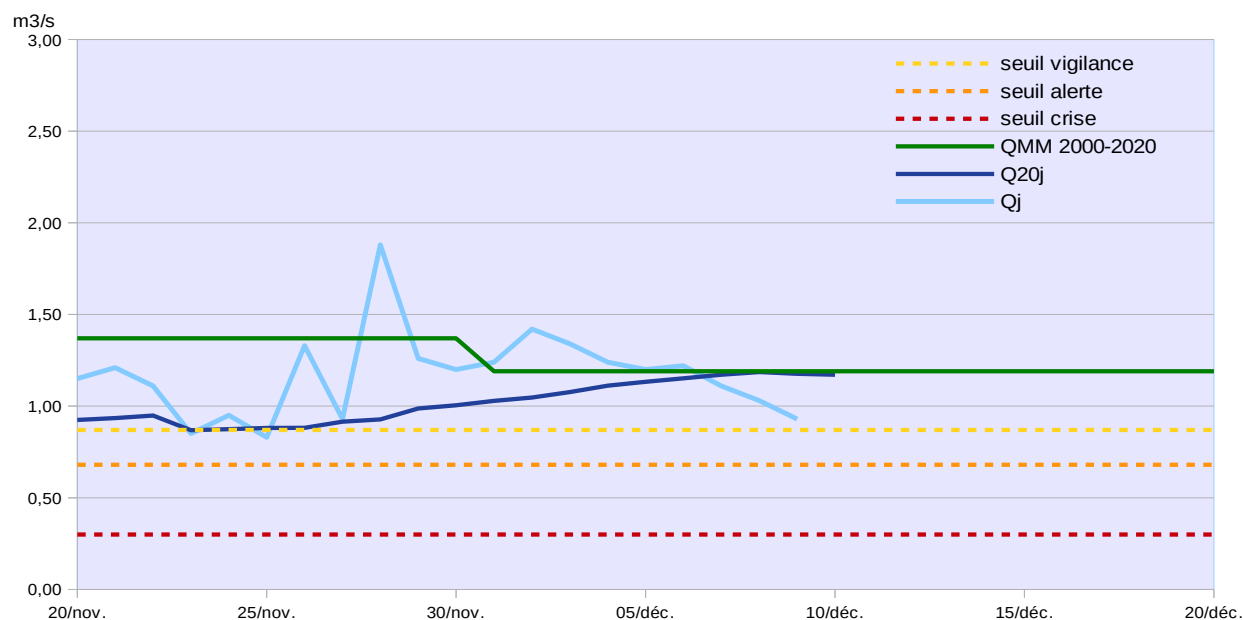
Courbe 3 : Variation du débit moyen sur 20 jours en 2024 sur la Rivière Moustique à Petit-Bourg
