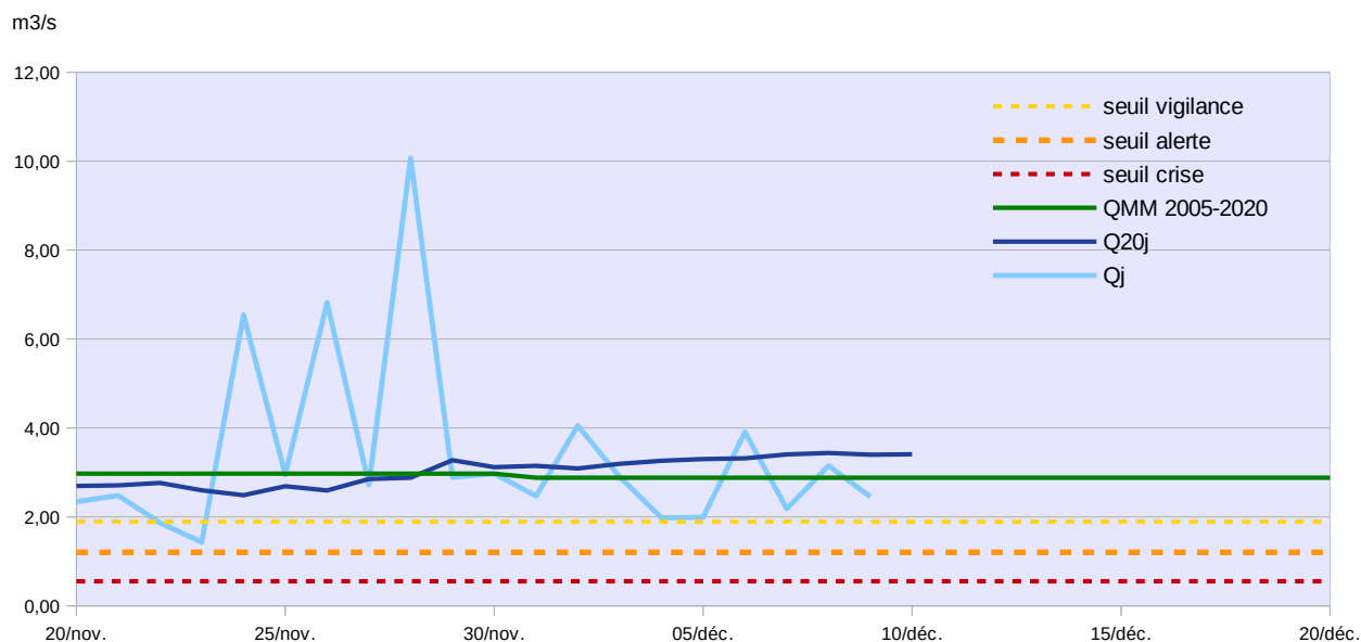
Courbe 2 : Variation du débit moyen sur 20 jours en 2024 sur la Grande Rivière de Capesterre
