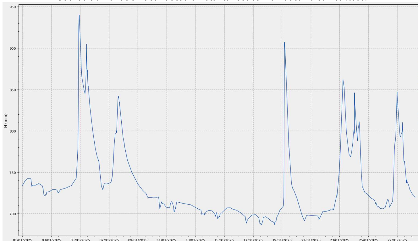
Courbe 6 : Variation des hauteurs instantanées sur La Boucan à Sainte-Rose.
