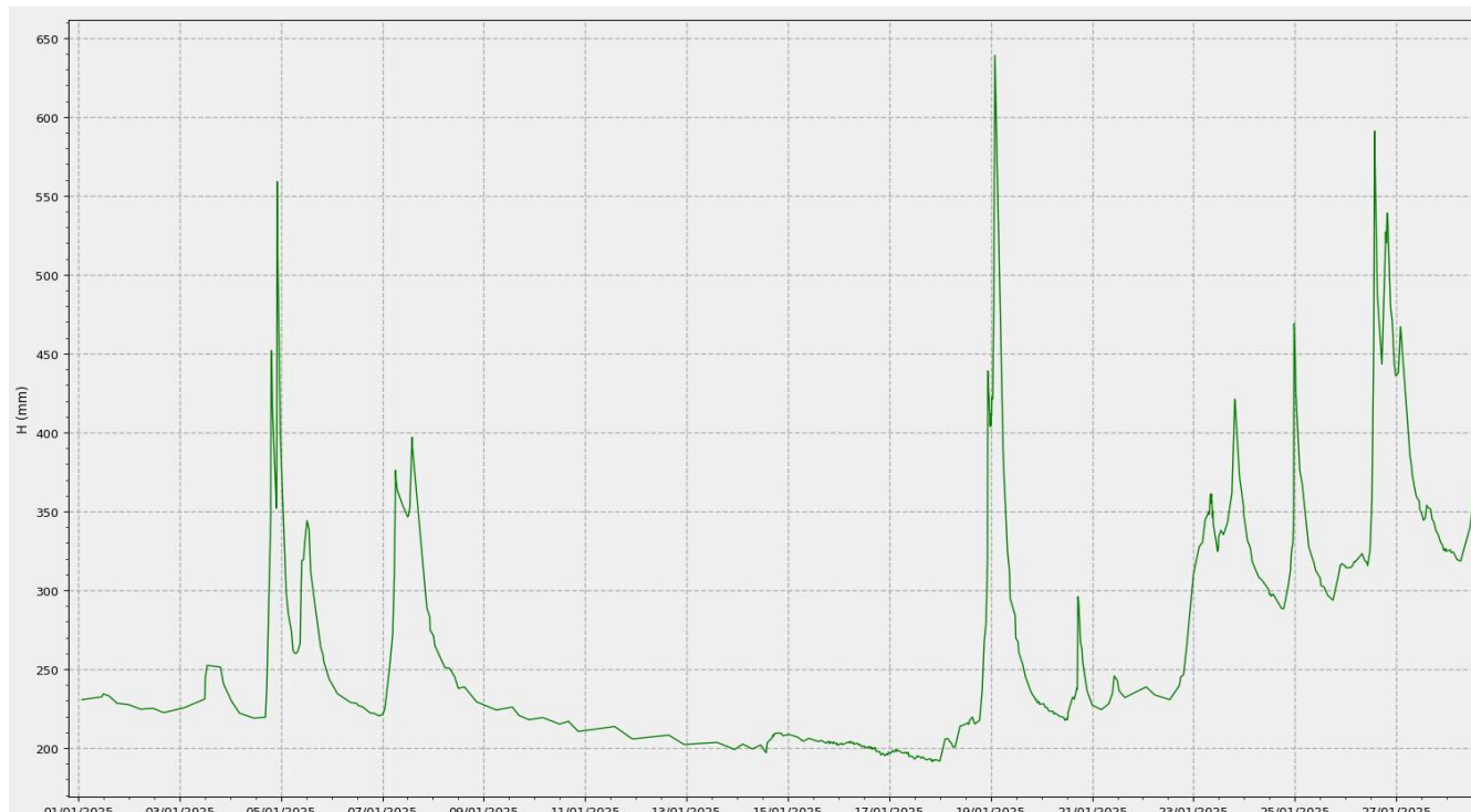
Courbe 5 : Variation des hauteurs instantanées sur Barthole à Vieux-Habitants
