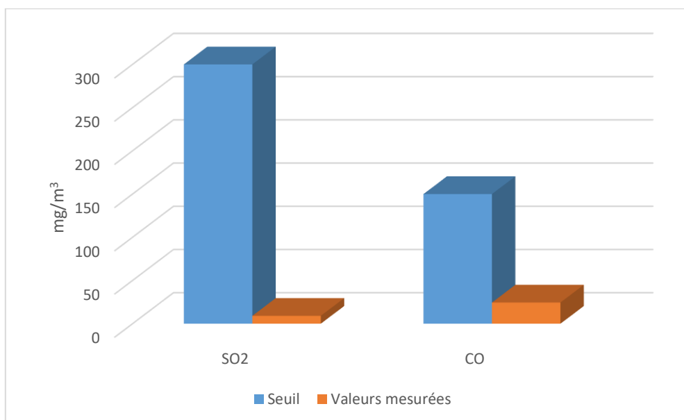
Figure 33 : Valeurs limites d'émissions torchère 2025
