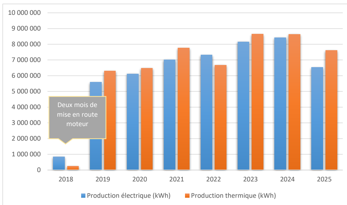
Figure 30 : Evolution de la production électrique et de la production thermique
