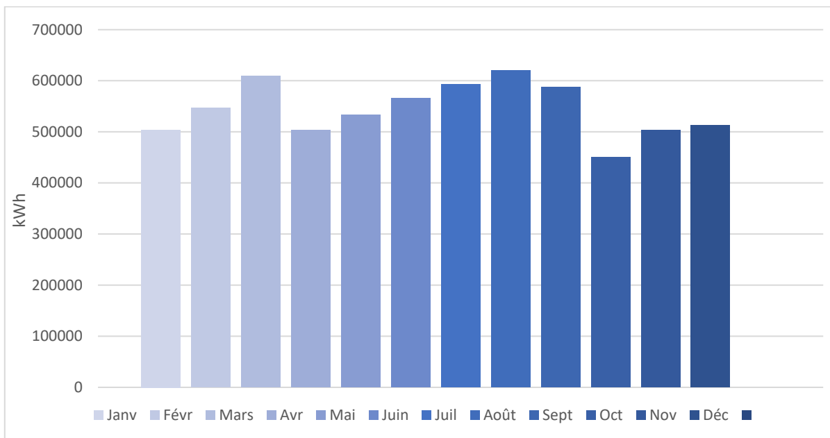
Figure 28 : Production électrique du moteur de valorisation du biogaz - 2025
