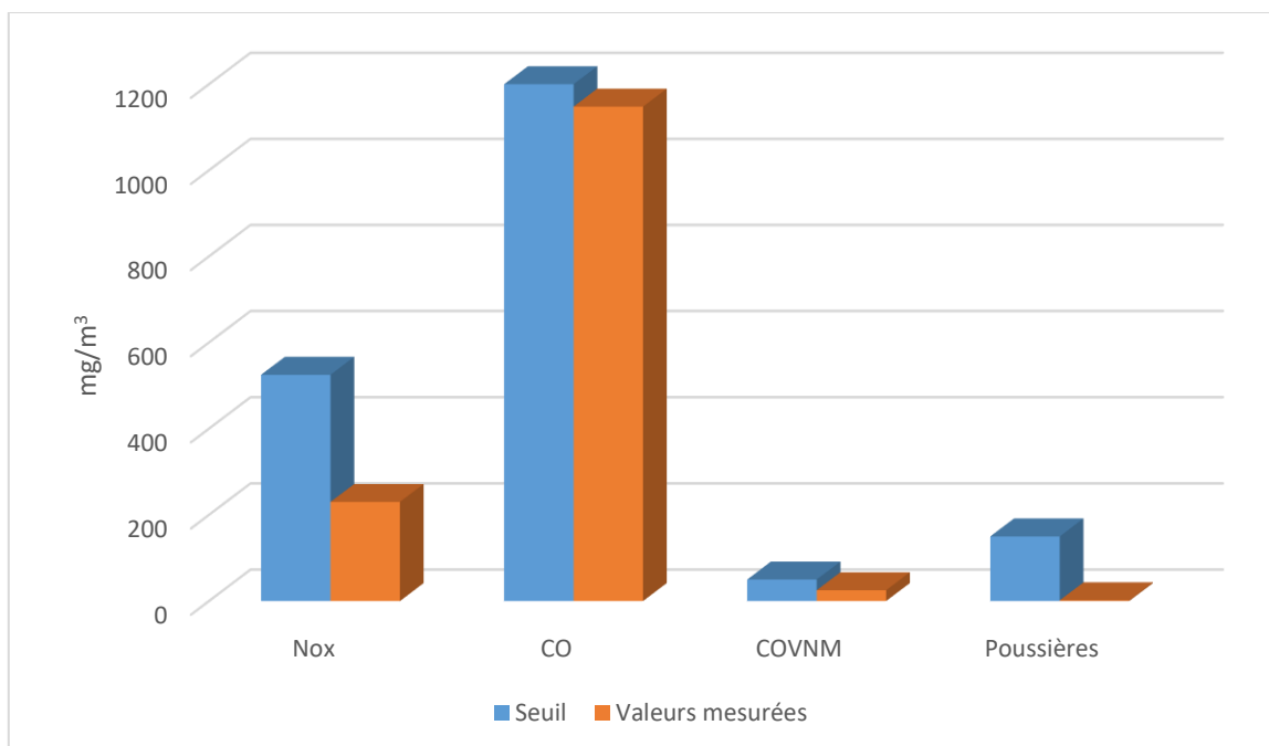
Figure 32 : Valeurs limites d'émissions moteur 2025
