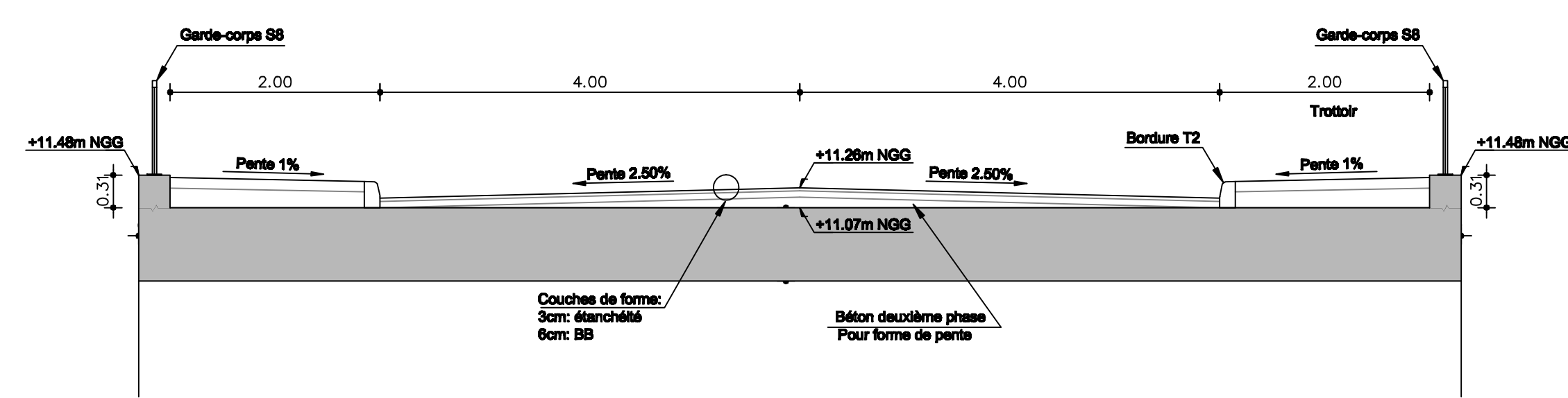
COUPE TYPE DE LA VOIRIE SUPERIEURE Echelle: 1/50
