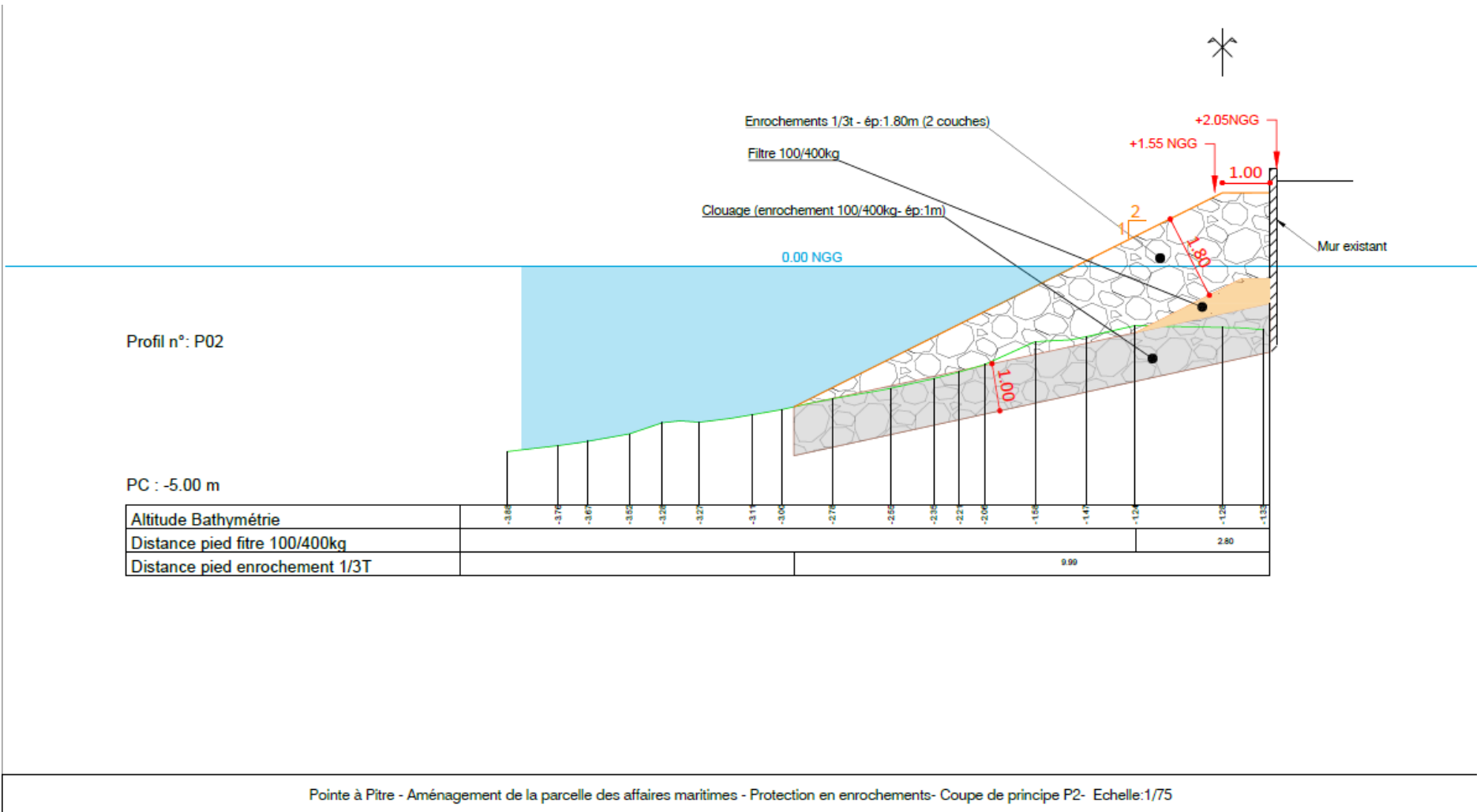
Coupe technique de principe – profil P2
