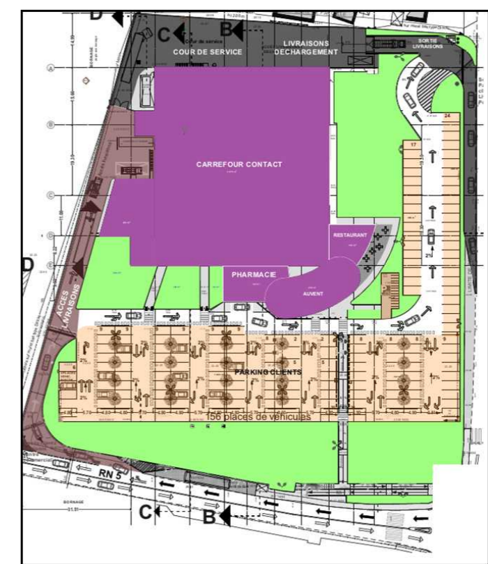
Plan masse de l'existant
