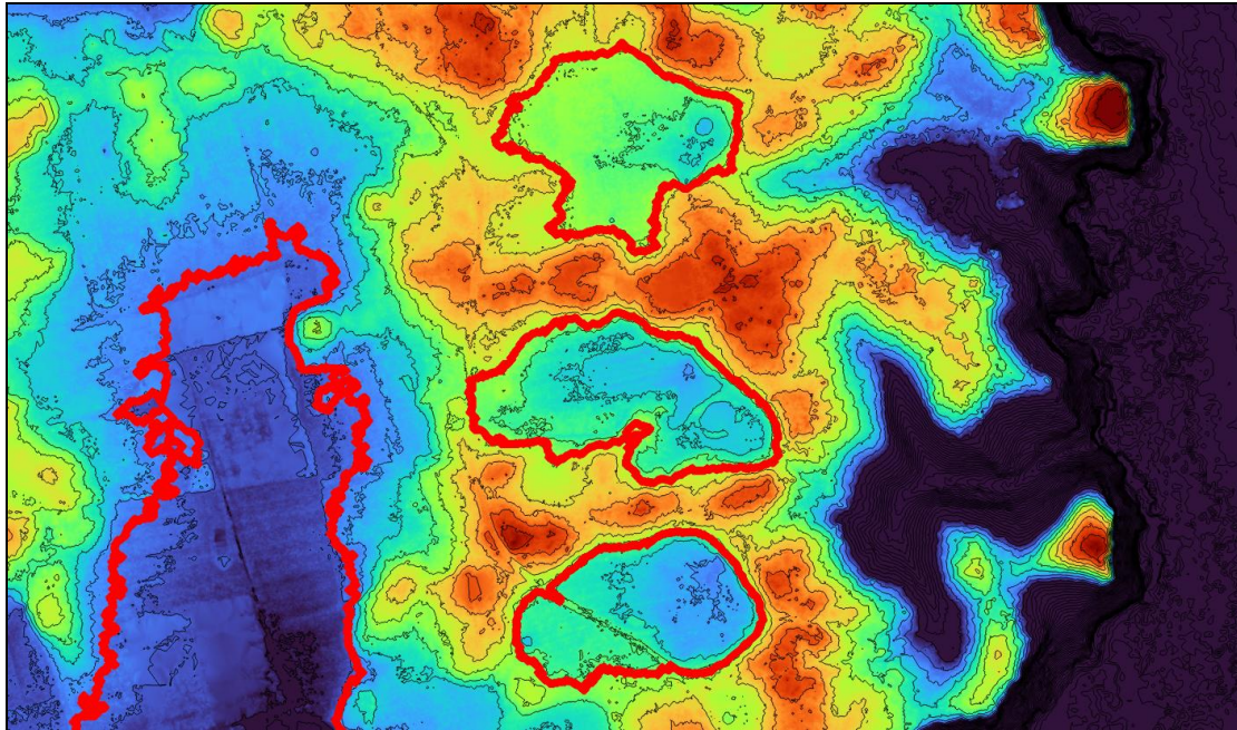
Figure 28 : Dépressions déconnectées du réseau hydrographique sur la commune de Petit-Canal [Source : Ginger CEBTP]
