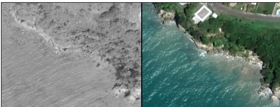
Figure 44 : Comparaison du littoral de Gosier entre les photos aériennes IGN de 1968 (à gauche) [Source : https://remonterletemps.ign.fr/ ] et les images satellite de 2022 (à droite) [Source : Google Earth]
