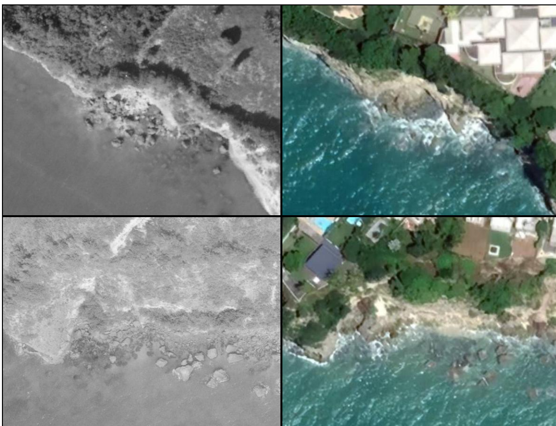
Figure 43 : Comparaison du littoral de Gosier entre les photos aériennes IGN de 1963 (en haut, à gauche), 1968 (en bas, à gauche) [Source : https://remonterletemps.ign.fr/ ] et les images satellite de 2022 (à droite) [Source : Google Earth]
