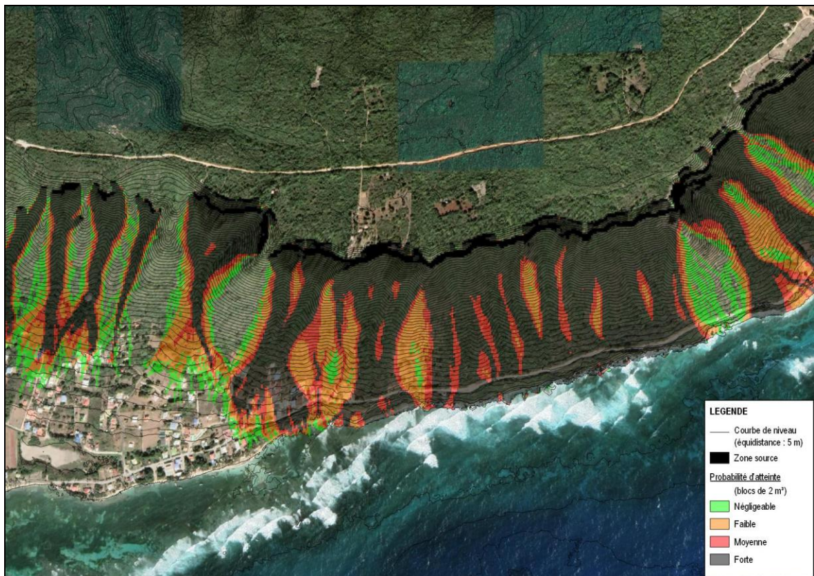
Figure 33 : Extrait des résultats de la modélisation trajectographique 3D (probabilité d'atteinte) sur La Désirade [Source : Ginger CEBTP]
