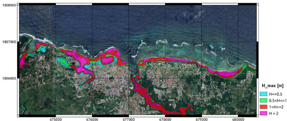
Figure 51 : scénario de référence à 2100 : extension de la submersion et hauteur d'eau maximale calculées sur la ville du Moule.
