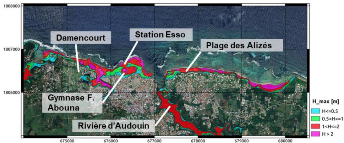
Figure 49 : Scénario de référence actuel : extension de la submersion et hauteur d'eau maximale calculées sur la Ville du Moule
