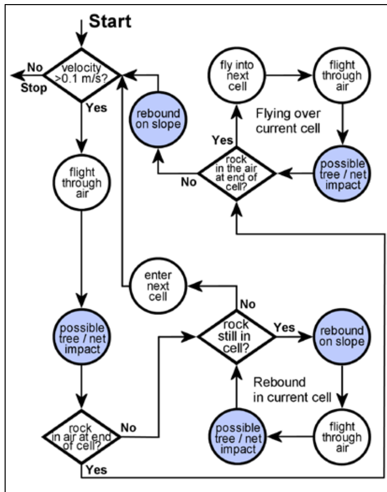
Figure 30 : Organigramme de Rockyfor3D. Les cercles colorés en bleu indiquent les étapes du modèle où des changements de direction sont susceptibles de se produire dans la chute du bloc simulé. [Source : Ecorisq]
