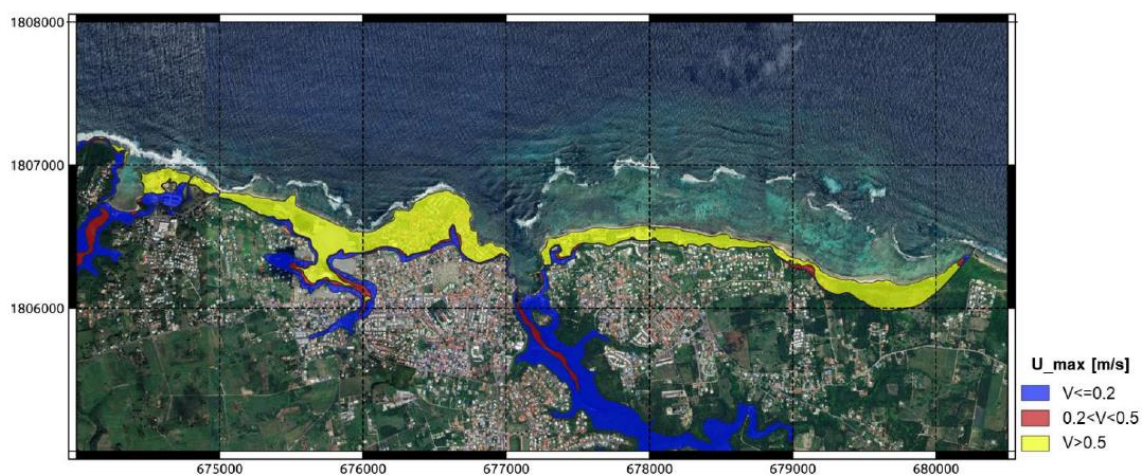
Figure 50 : Scénario de référence actuel : vitesse maximale des courants moyennées calculées sur la ville du Moule
