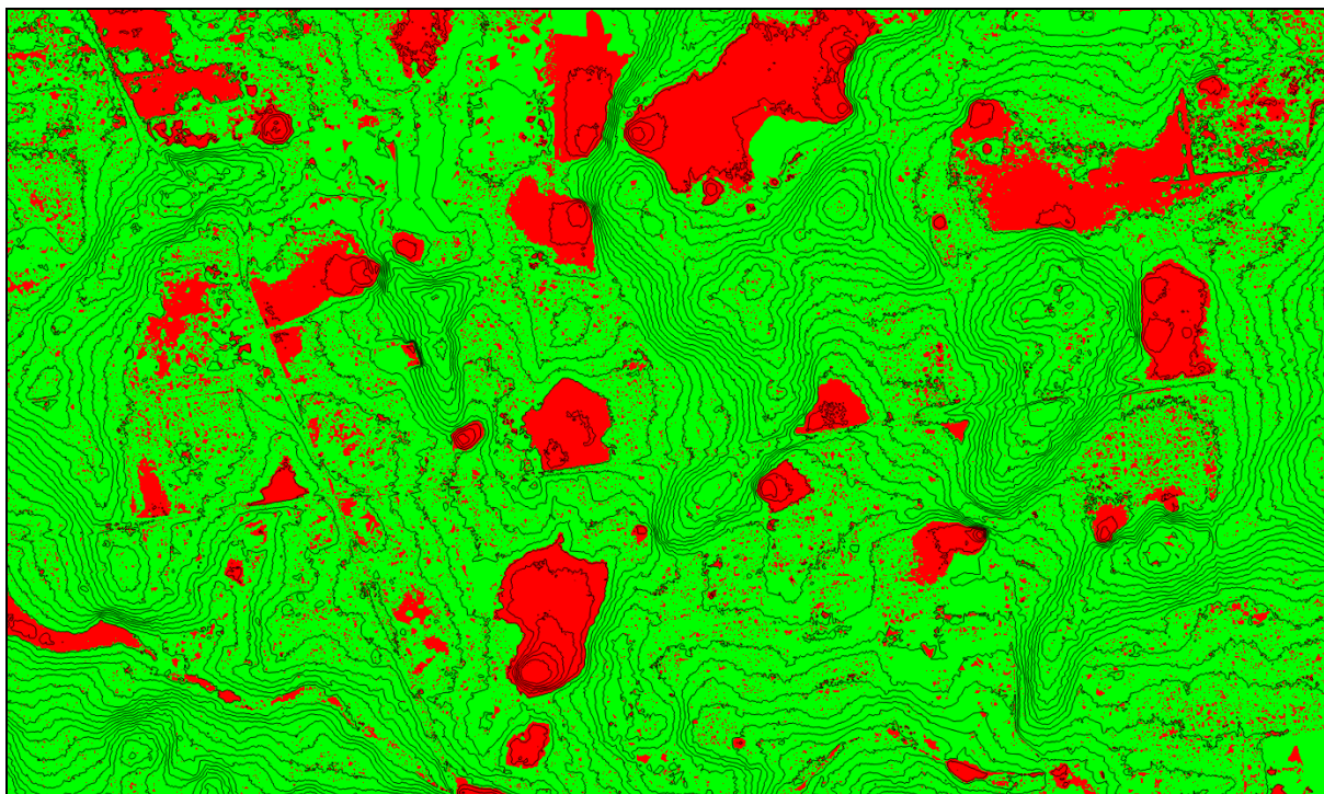
Figure 26 : Détection des dépressions (en rouge) avec l'outil StochasticDepressionAnalysis de WhiteboxTools sur la commune de Petit-Canal [Source : Ginger CEBTP]
