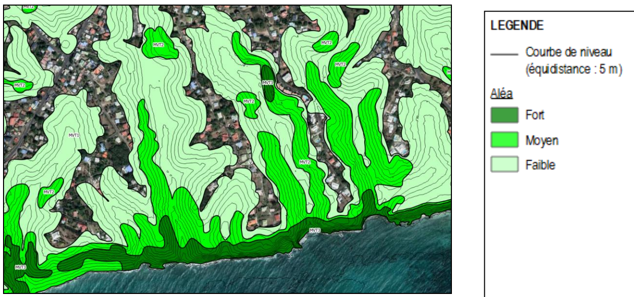
Figure 46 : Extrait de l'aléa Mouvements de terrain finalisé sur la commune du Gosier [Source : Ginger CEBTP]
