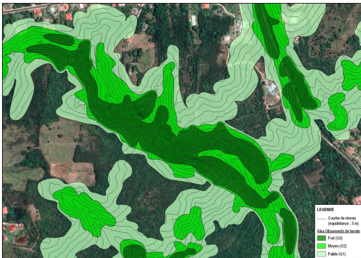
Figure 37 : Extrait de l'aléa Glissements de terrain finalisé sur Marie-Galante [Source : Ginger CEBTP]
