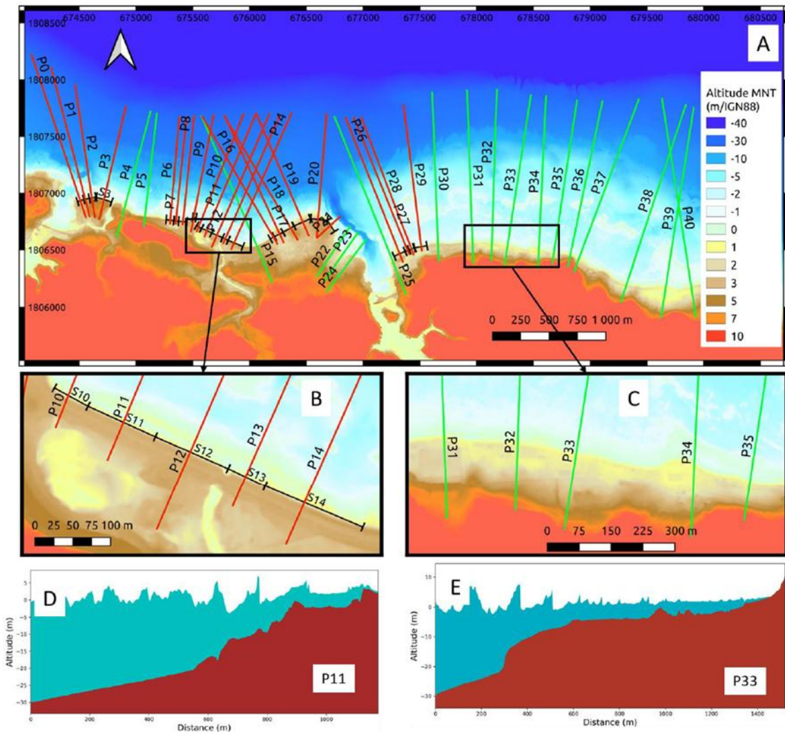
Figure 48 : implantation des profils sur le site du Moule pour le calcul de la submersion et des débits franchissant avec SWAS. A : Vue de l'ensemble des 41 profils ; B : exemple de profils à franchissements ; C : exemple de profils pour le calcul de la submersion
