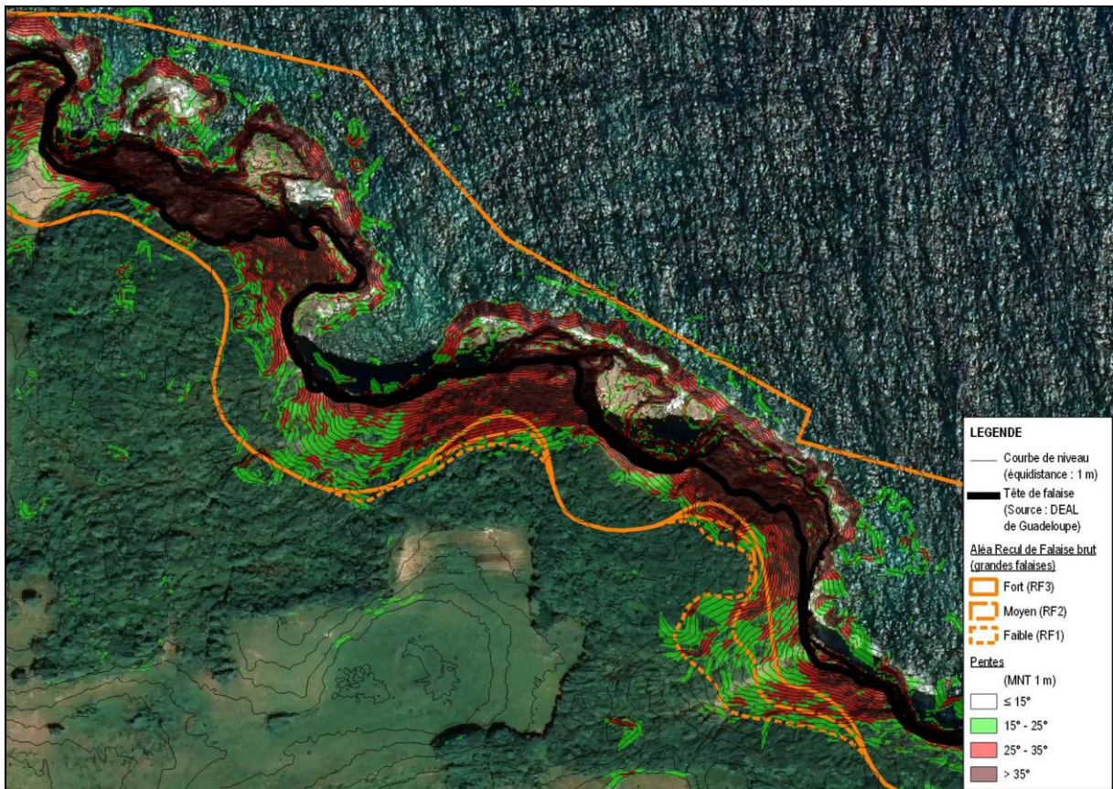
Figure 40 : Extrait de la saisie manuelle de l'aléa Recul de Falaise brut (grandes falaises) sur Marie-Galante [Source : Ginger CEBTP]
