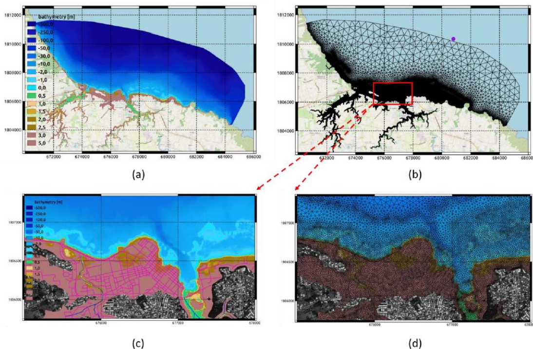
Figure 47 : Site du Moule : (a) : emprise spatiale du domaine de calcul et données topo-bathymétriques ; (b) Maillage de calcul et point de forçage (en violet) ; (c) topo-bathymétrie et lignes de contraintes (violet et bleu) dans la ville du Moule ; (d) zoom du m
