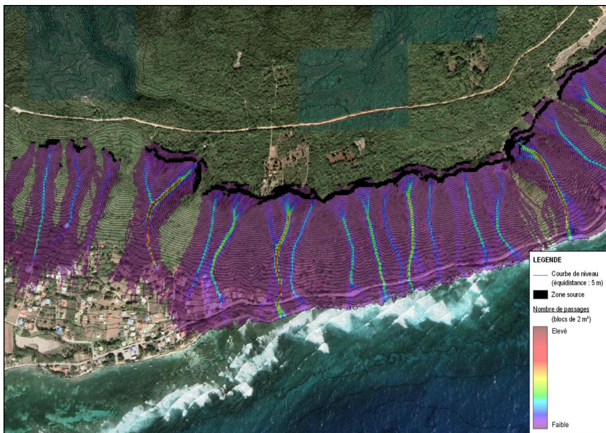
Figure 31 : Extrait des résultats de la modélisation trajectographique 3D (nombre de passages) sur La Désirade [Source : Ginger CEBTP]
