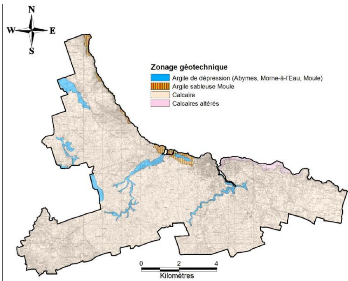
Figure 5 : Zonage géotechnique [Source : rapport BRGM/RP-61989-FR]
