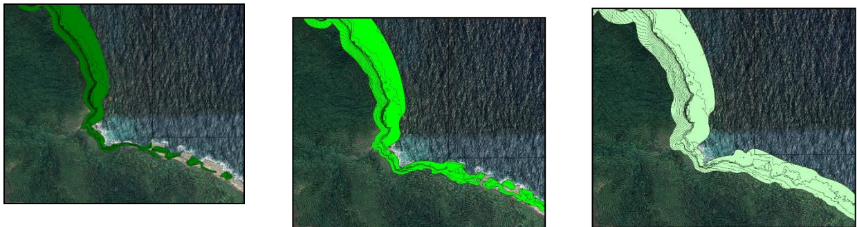
Figure 41 : Extraits des aléas Recul de Falaise Fort assemblés (à gauche), Moyen (au centre) et Faible (à droite) avec tampons et lissée sur Marie-Galante [Source : Ginger CEBTP]
