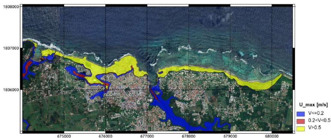
Figure 52 : Scénario de référence à 2100 : vitesse maximale des courants moyennés calculés sur la ville du Moule.
