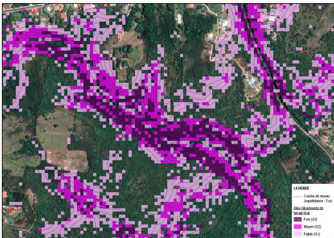
Figure 35 : Extrait de l'aléa Glissements de terrain brut sur Marie-Galante [Source : Ginger CEBTP]
