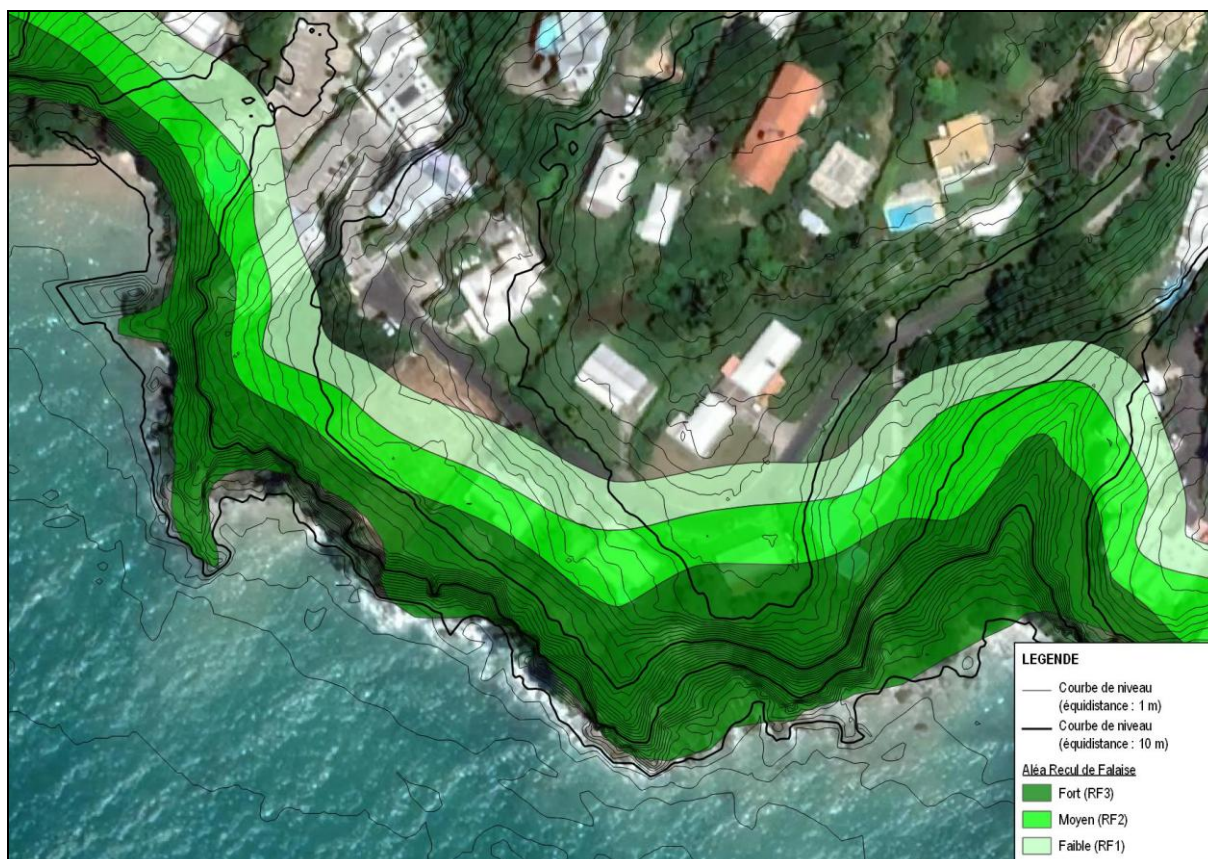
Figure 45 : Extrait de l'aléa Recul de Falaise sur une zone à enjeux forts à Gosier sur Grande-Terre [Source : Ginger CEBTP]
