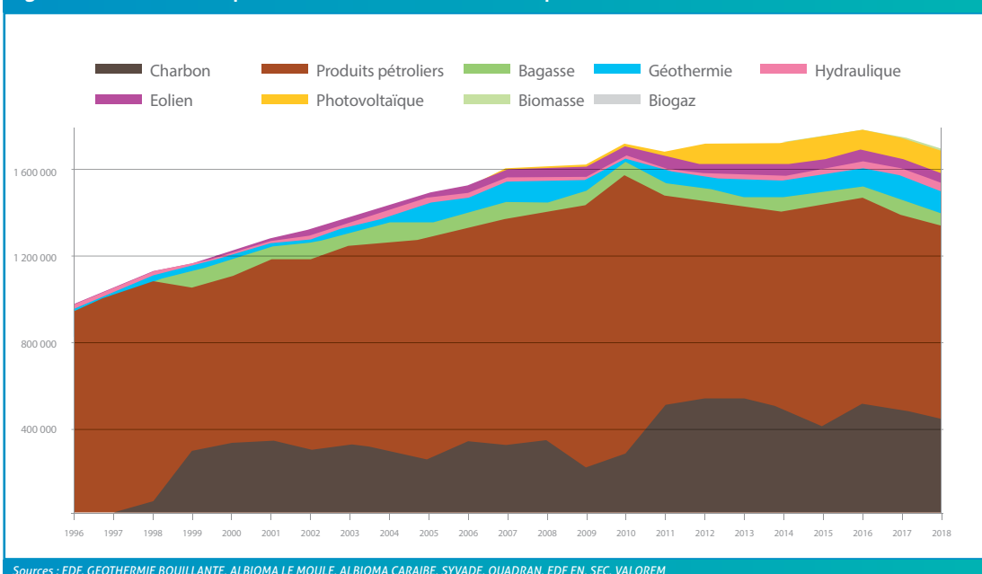
Figure 16 : Evolution de la production d'électricité en Guadeloupe
