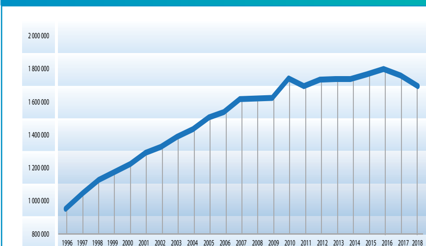
Figure 4 : Consommation d'électricité à partir de 1996, en GWh.
